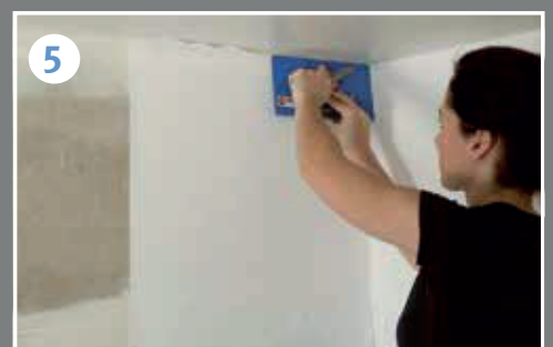
5 Überstände mit einem Kunststoffspachtel in die Ecke drücken und mit einem Cutter-Messer beschneiden.
